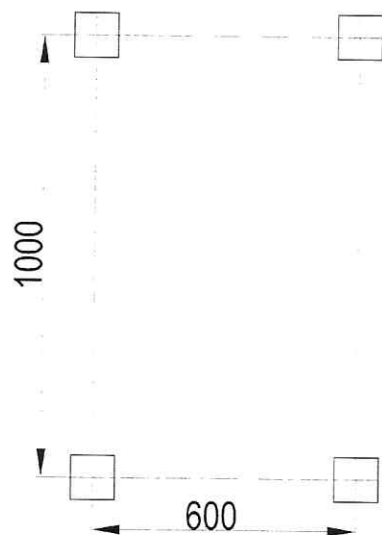
Схема расположения фундаментов
