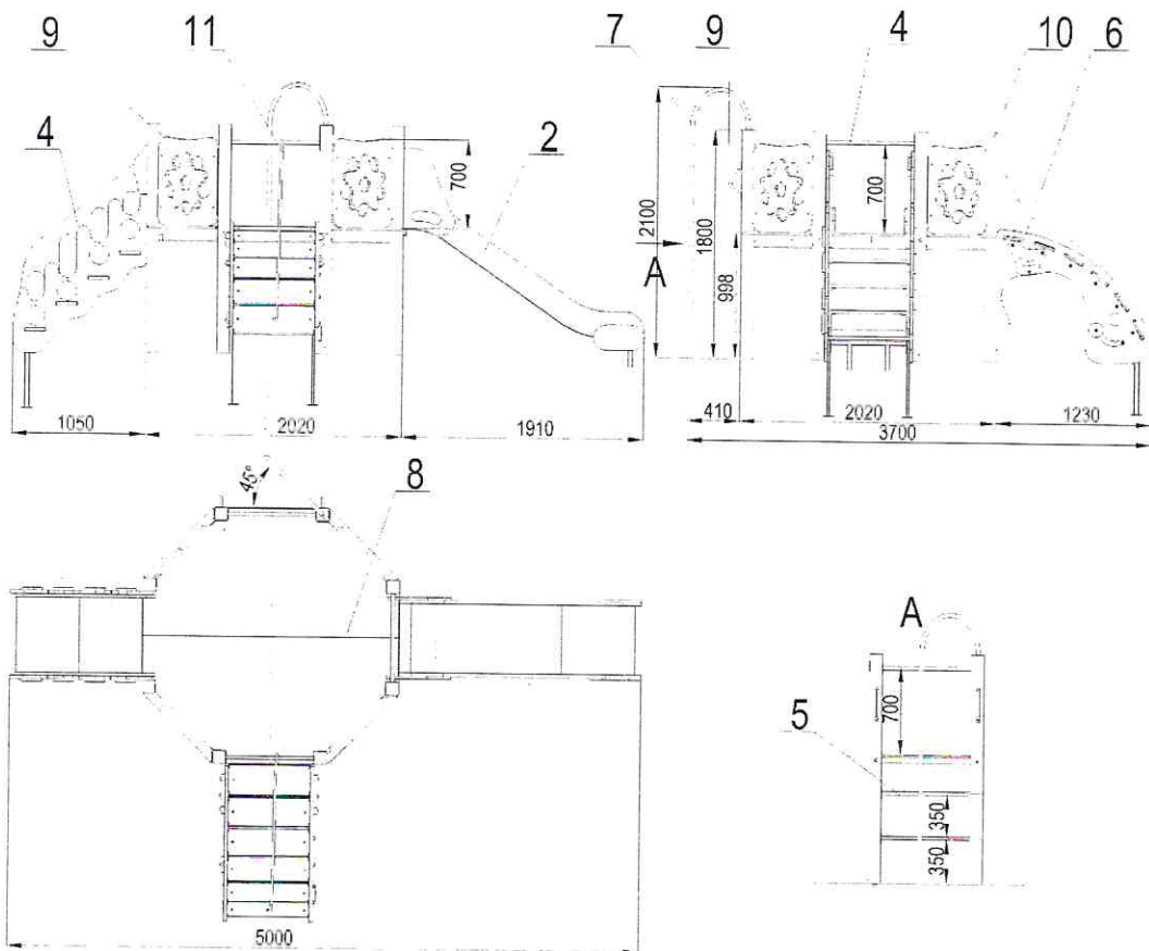
Общий вид детского игрового оборудования.
