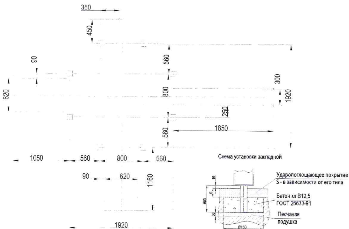
Схема расположения фундаментов
