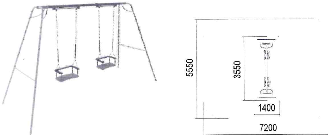
Общий вид детского игрового оборудования.
