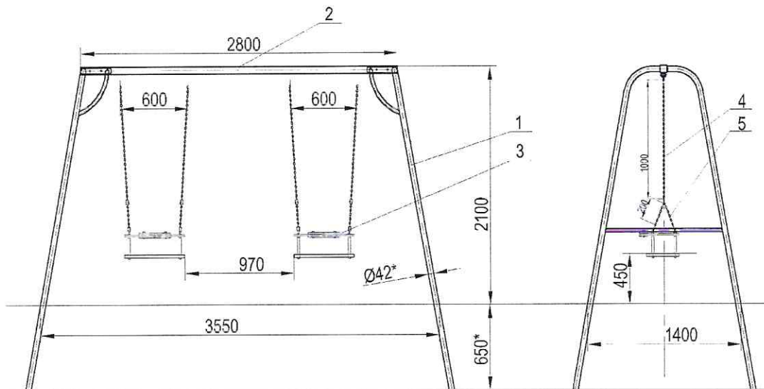
Общий вид детского игрового оборудования.
