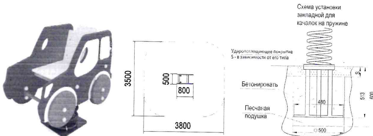
Общий вид детского игрового оборудования.
