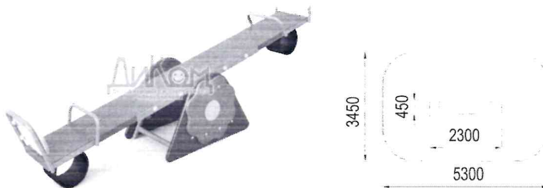
Общий вид детского игрового оборудования.
