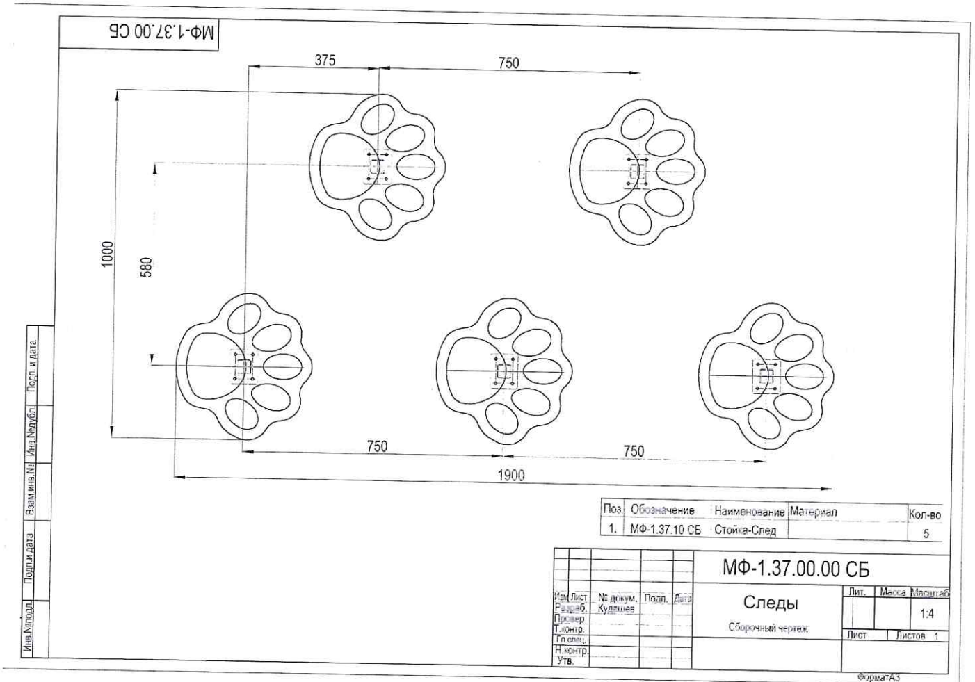
Общий вид детского игрового оборудования.
